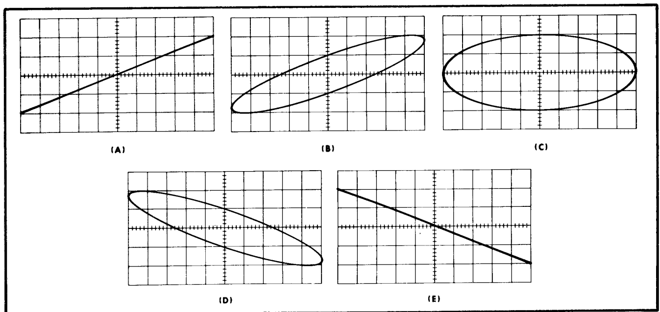
Fig. 2-27. Phase of lissajous display. (A) 0° or 360°, (B) 30° or 330°, (C) 90° or 270°, (D) 150° or 210° and (E) 180°.
